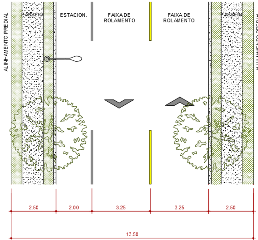
PLANTA VIA LOCAL
