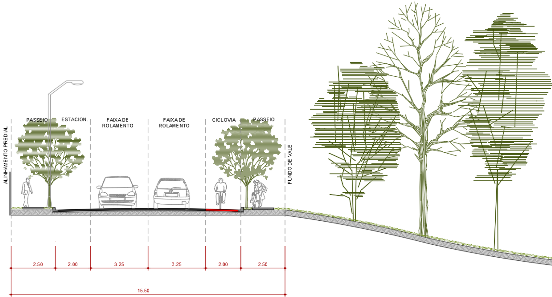
PERFIL VIA MARGINAL DE APP
