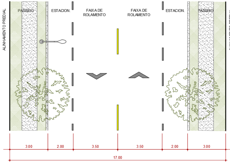
PLANTA VIA COLETORA
