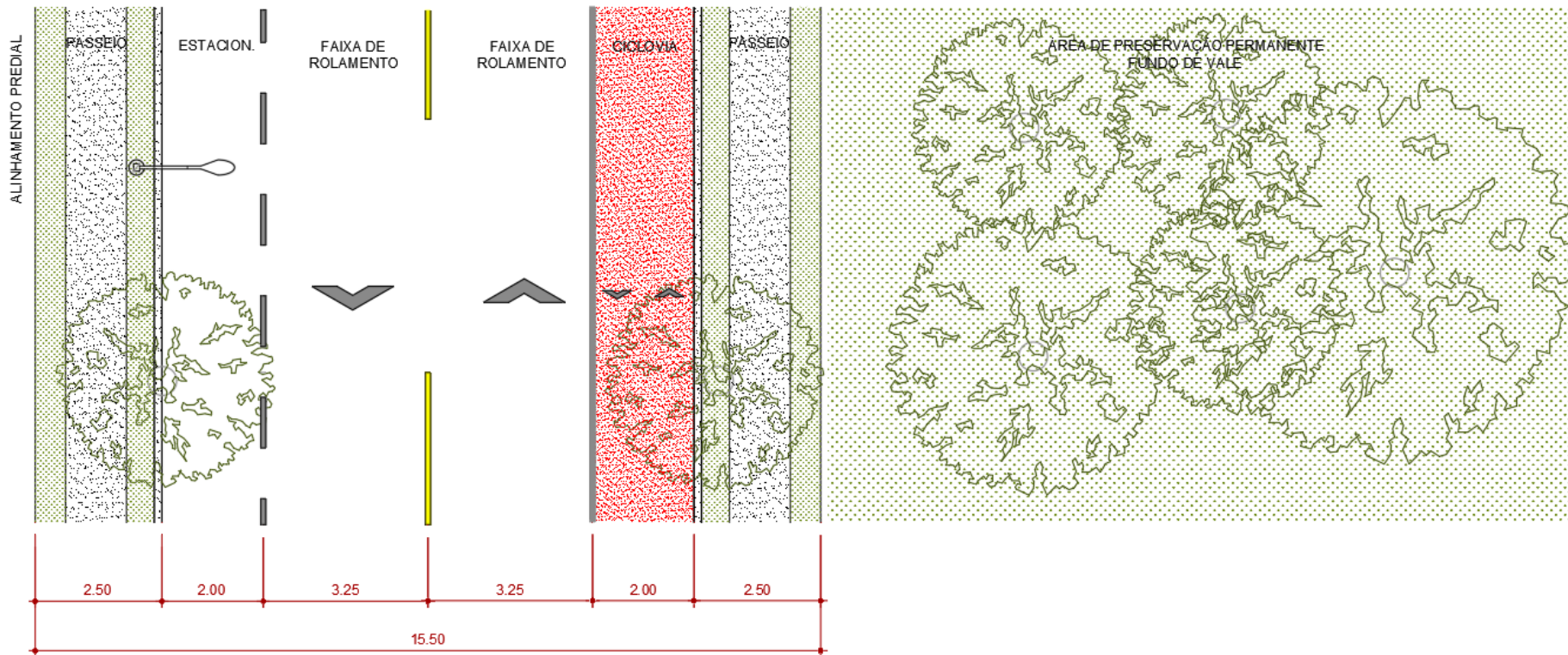
PLANTA VIA MARGINAL DE APP
