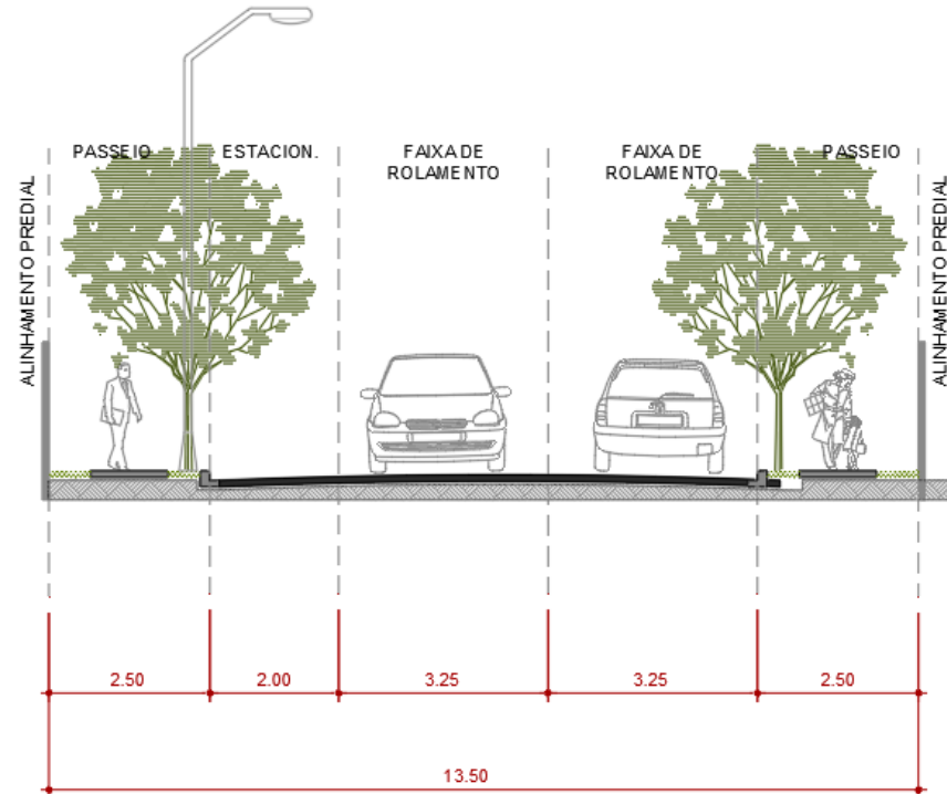
PERFIL VIA LOCAL
